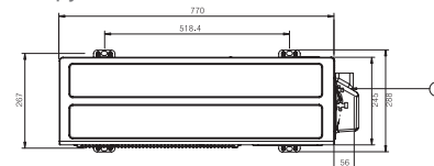
Наружный блок
